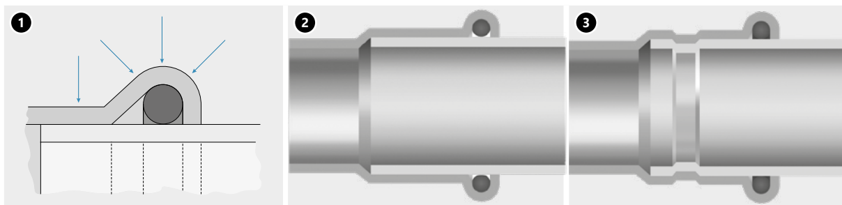
1. Press kötésben nyomás iránya. 2. Kötés metszete préselés előtt. 3. Kötés metszete préselés után.
