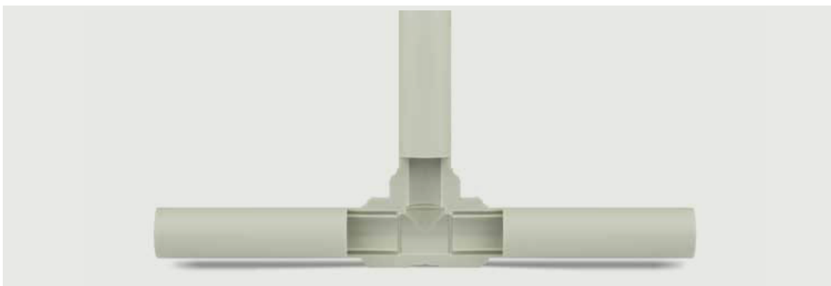
Hegesztett kötés keresztmetszete
