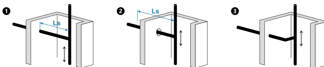
Rugalmas kar a felszálló vezeték elágazásai a csővezető csatornában (példa)
