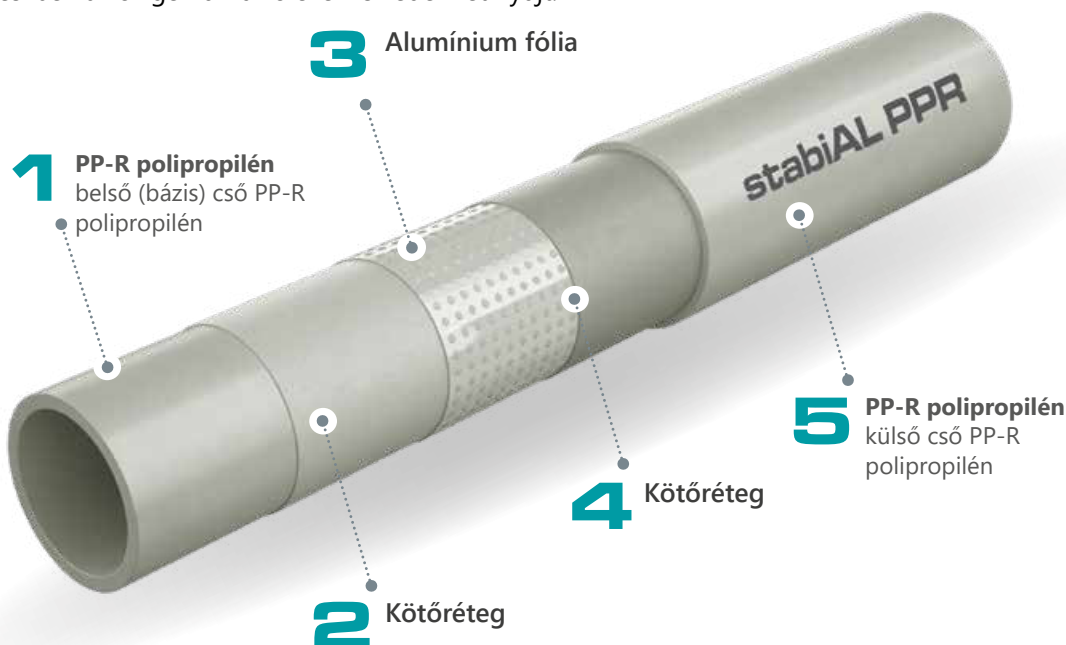
KAN-therm PP stabiAL PPR kompozit cső szerkezete
