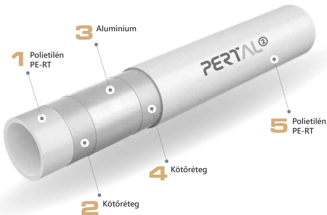
PERTAL 2 cső keresztmetszete
