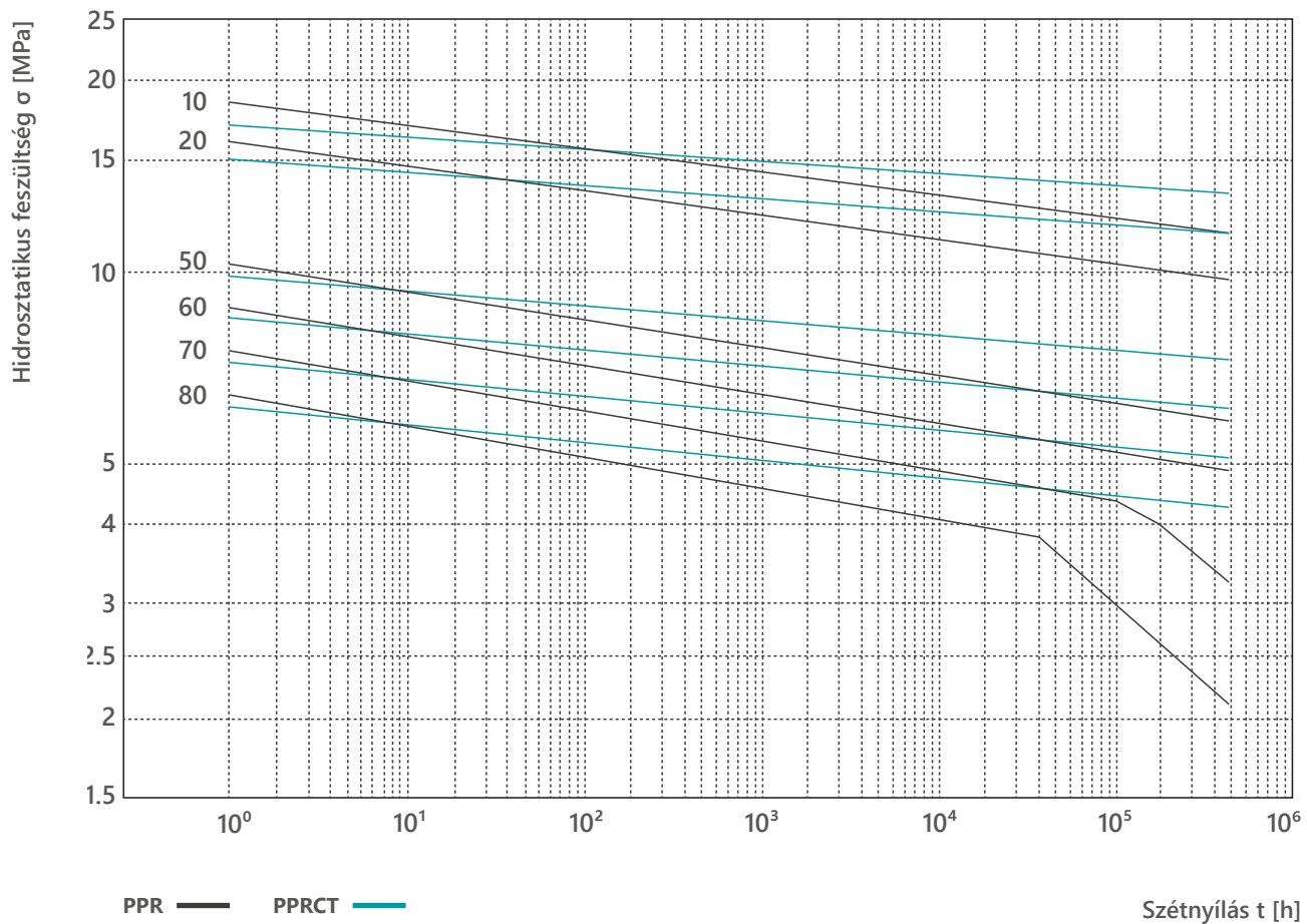
Diagram PPR és PPRCT csövekre ( t=[10-80]^{\circ}\text{C} )
