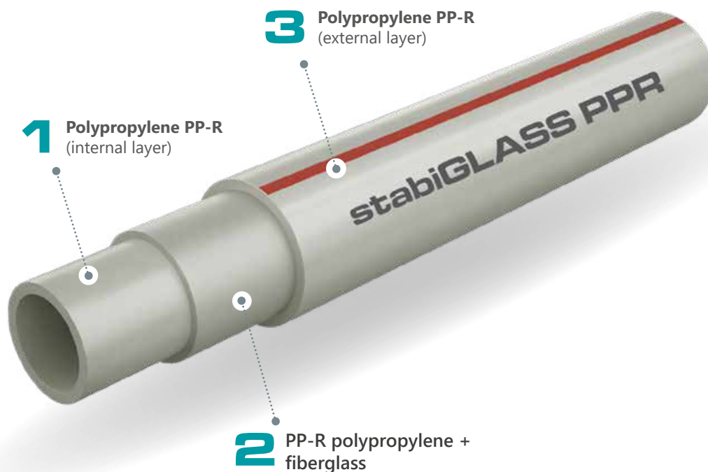
KAN-therm PP stabiGLASS PPR cső szerkezete
