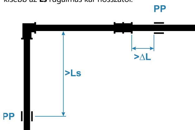
Csúszó pontok megfelelő elhelyezése L_s – rugalmas kar hossza, \Delta L – a csőszakasz max. tágulása)
