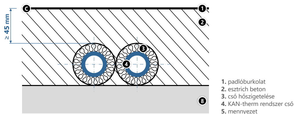
C. Közvetlen az esztrich betonban
