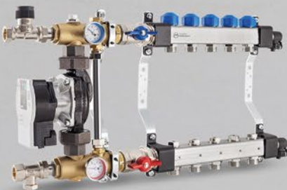
Osztó-gyűjtő szabályzó és keverő szelepekkel, fűtőköri keverőegységgel Wilo Para 25/6 szivattyú - USVP sorozat
