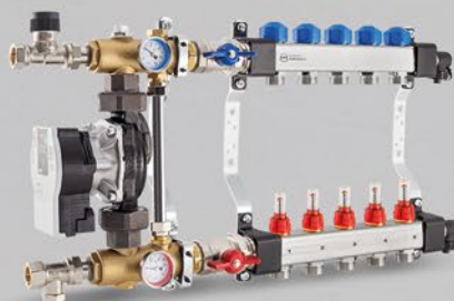
Osztó-gyűjtő térfogatáram mérővel és keverő szelepekkel, fűtőköri keverőegységgel Wilo Para 25/6 szivattyú - USFP sorozat
